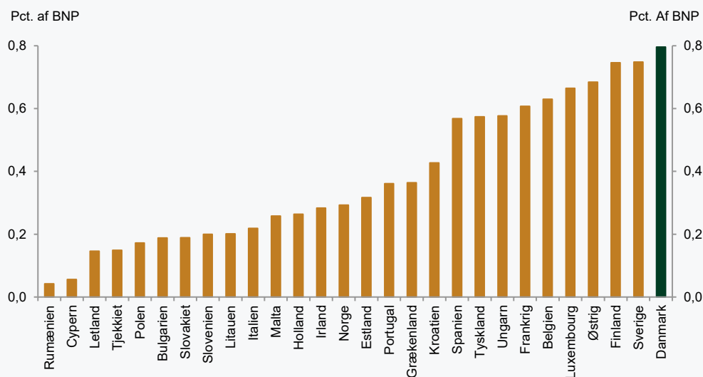
Figur 7.3. Udgifter til den aktive beskæftigelsesindsats på tværs af lande, 2019
